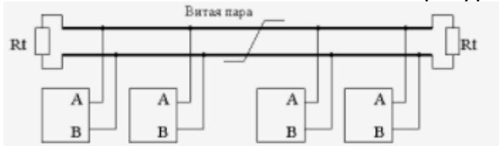
Рис. 10. Схема согласования и конфигурации линии связи А и В.
