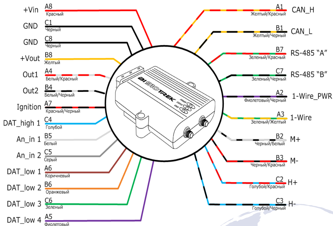
Рис. 4. Назначение контактов BI 920 TREK
