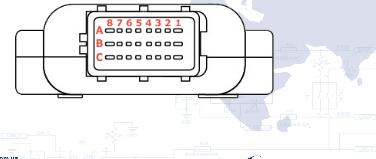
Рис. 3. Расположение разъёма и нумерация контактов
