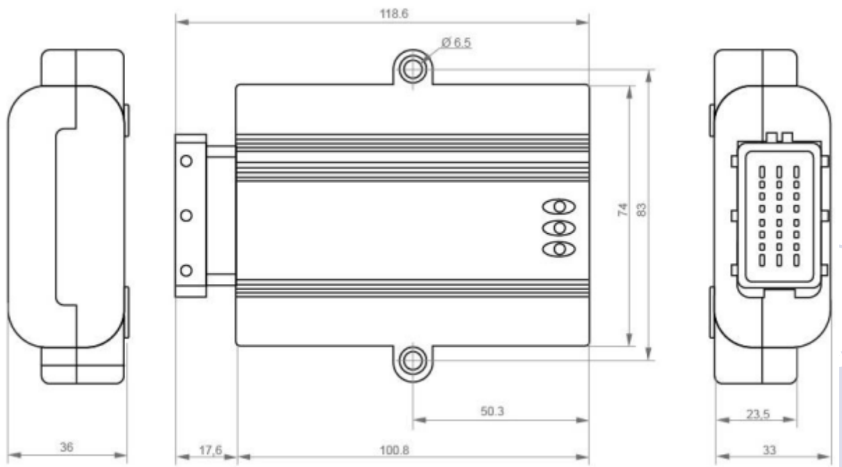
Рис. 2. Внешний вид и габаритные размеры устройства наблюдения «VI 920 TREK». (Вид сзади)
